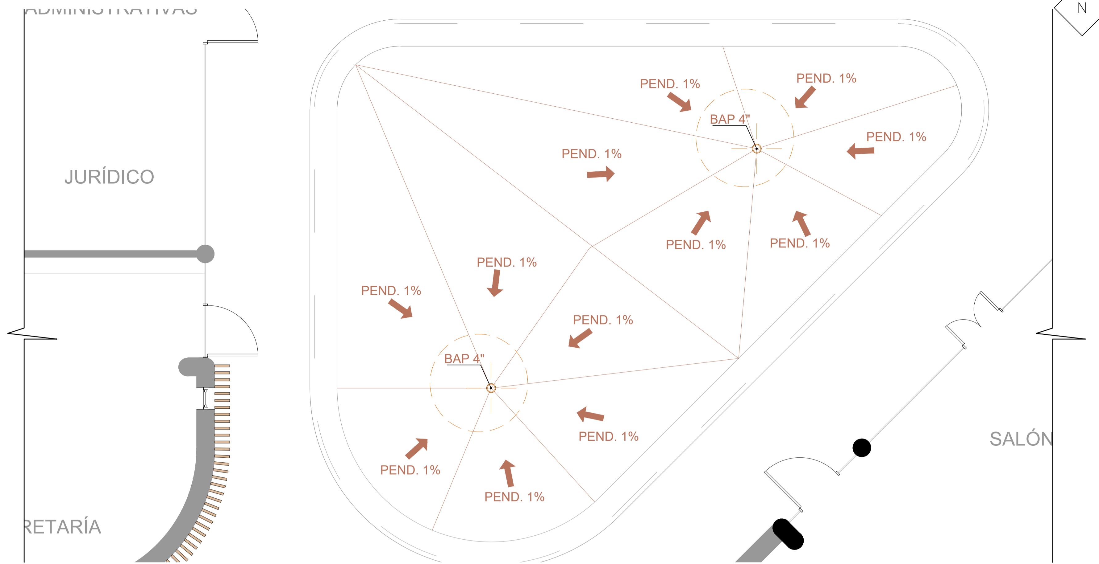
AMPLIACIÓN #1 DRENAJES PLUVIALES ESCALA 1: 50
