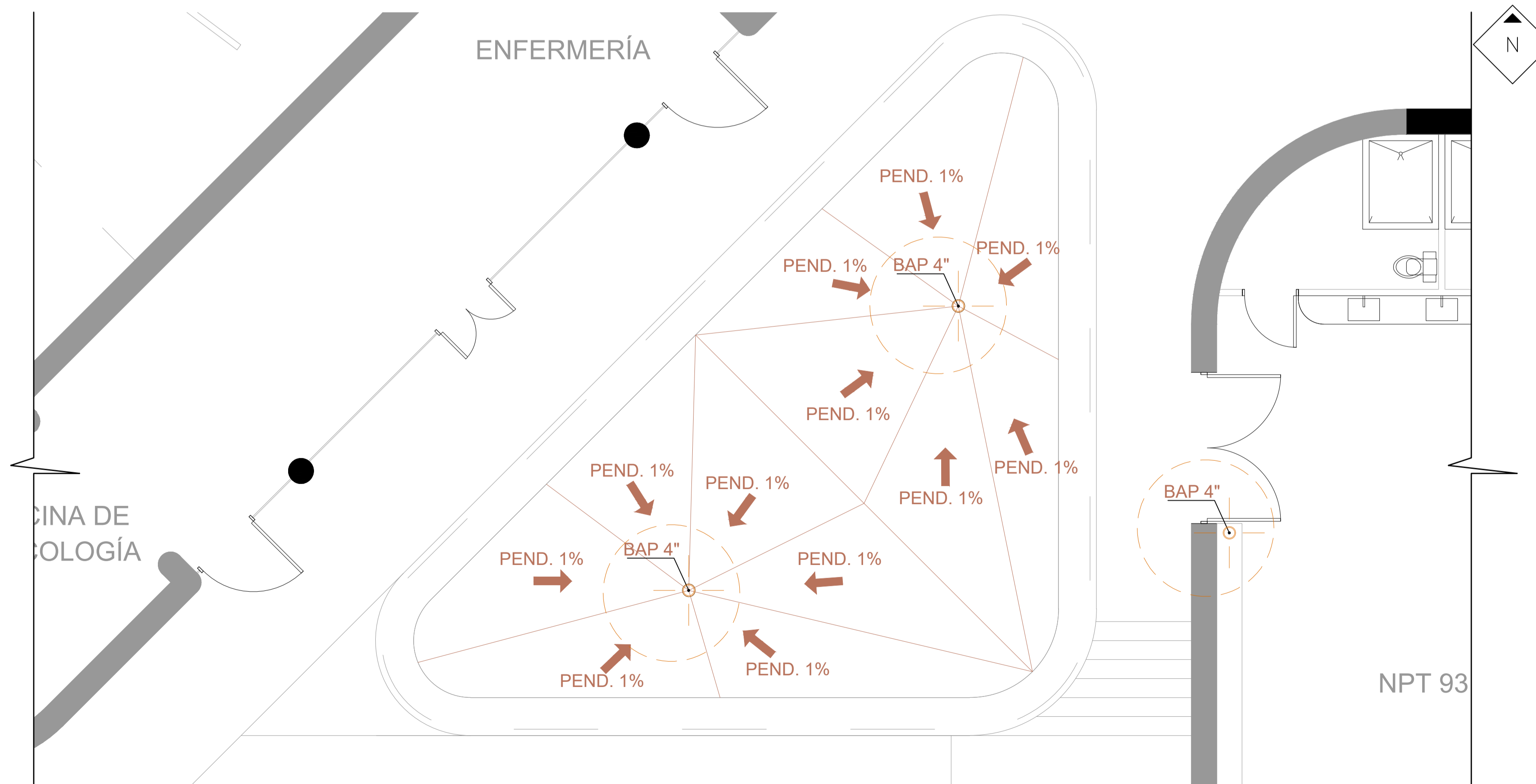
AMPLIACIÓN #2 DRENAJES PLUVIALES ESCALA 1: 50
